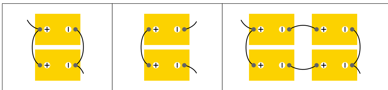
Параллельное соединение
