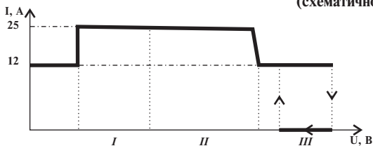
Вольт-Амперная характеристика работы Вымпел-410 (схематично)
